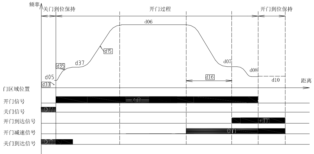
图 7：开门运行曲线图
