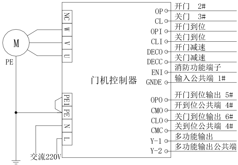
图2：控制器接线图
