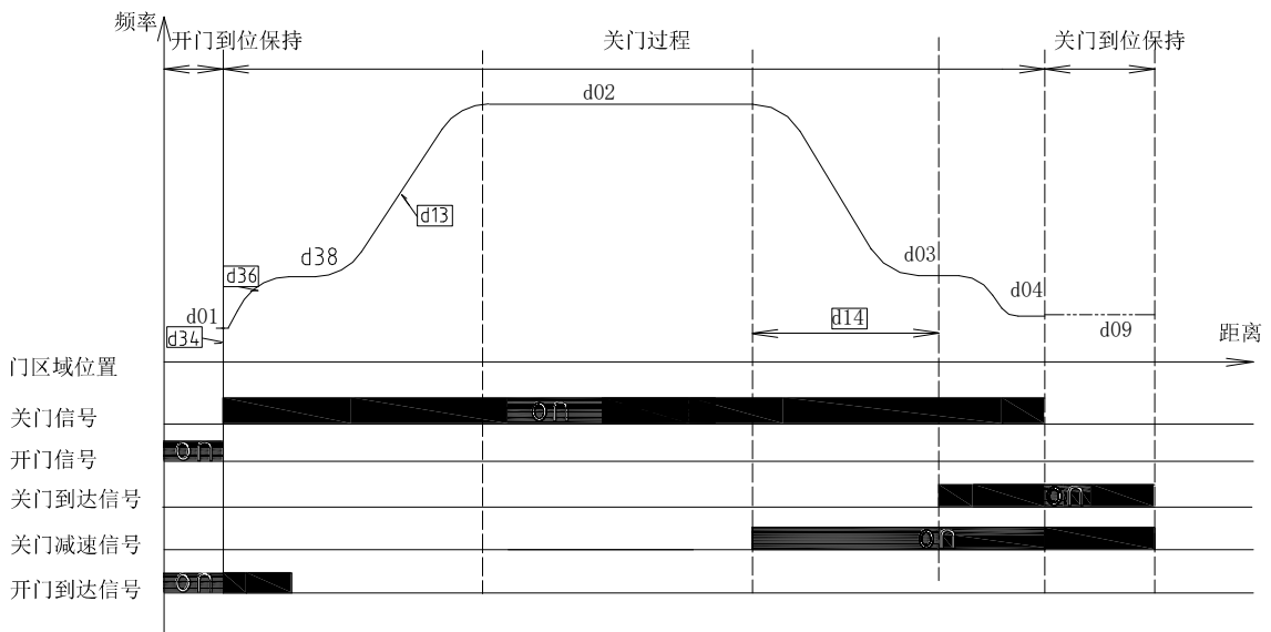
图 8：关门运行曲线图
