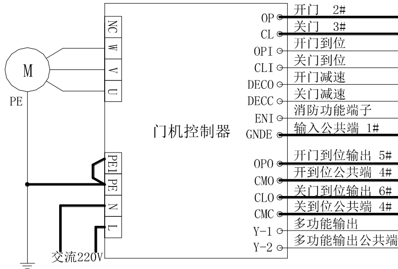
图3：控制器接线确认图
